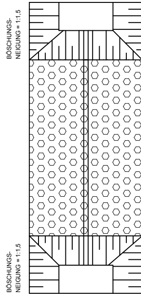
GRUNDRISS
