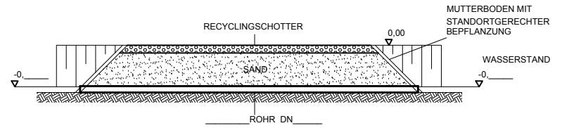
LÄNGSSCHNITT
