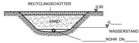
QUERSCHNITT
